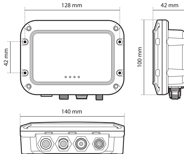
Abbildung 5 AIS-Transponder Abmessungen
