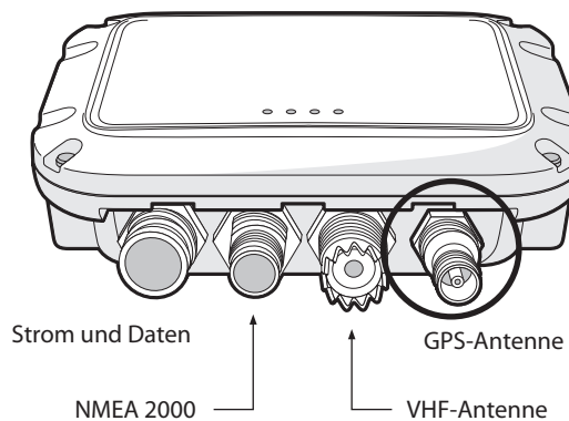
Abbildung 8 Position des GPS-Antennensteckverbinders
