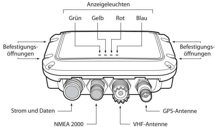
Abbildung 2 AIS-Transponder-Übersicht
