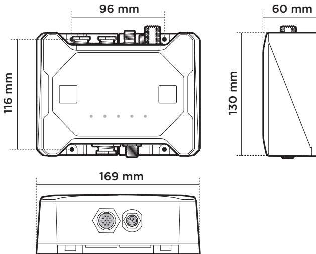
Figuur 2 Afmetingen van transponder
