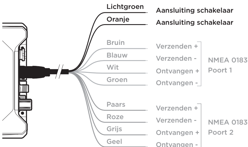
Figuur 19 Een externe schakelaar aansluiten
