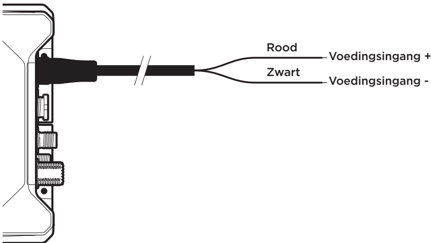
Figuur 9 De voedingsbron aansluiten
