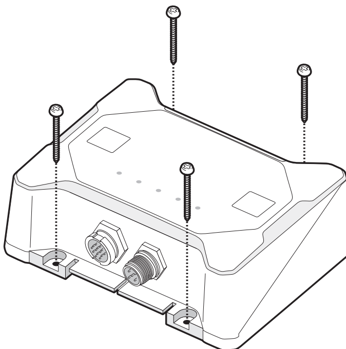
Figuur 11 Installatie van de AIS transceiver
